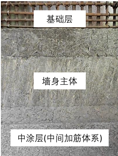
土墙的结构
