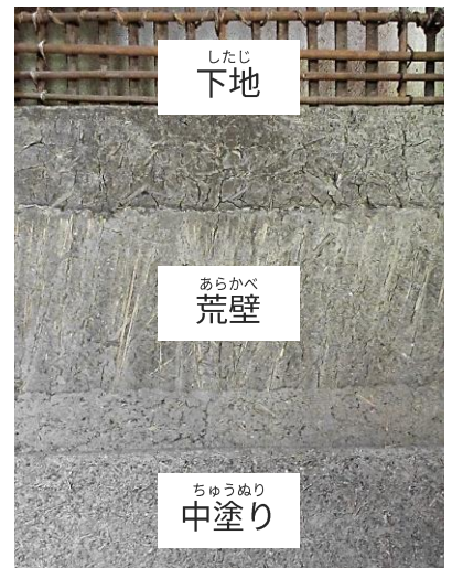
土壁の構造
