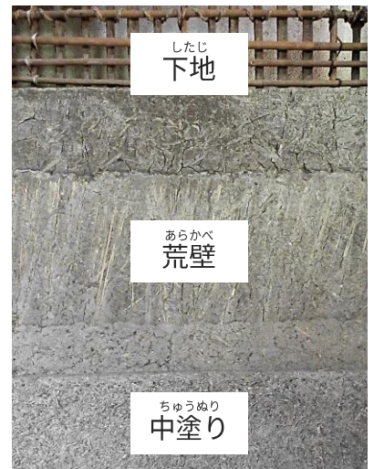
土壁の構造
